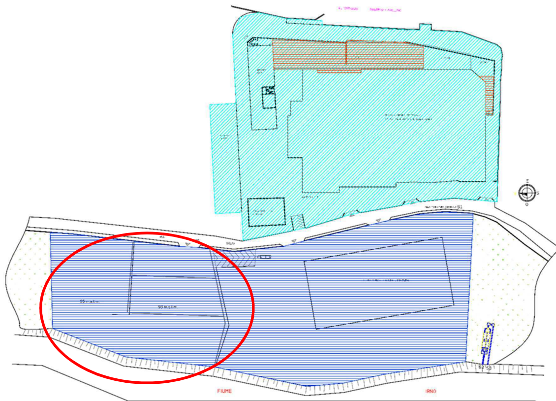
Figura 12 - Stralcio planimetrico
