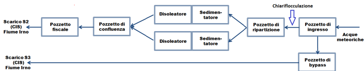
Figura 3 - Schema a blocchi impianto di trattamento acque di prima pioggia - STATO ATTUALE
