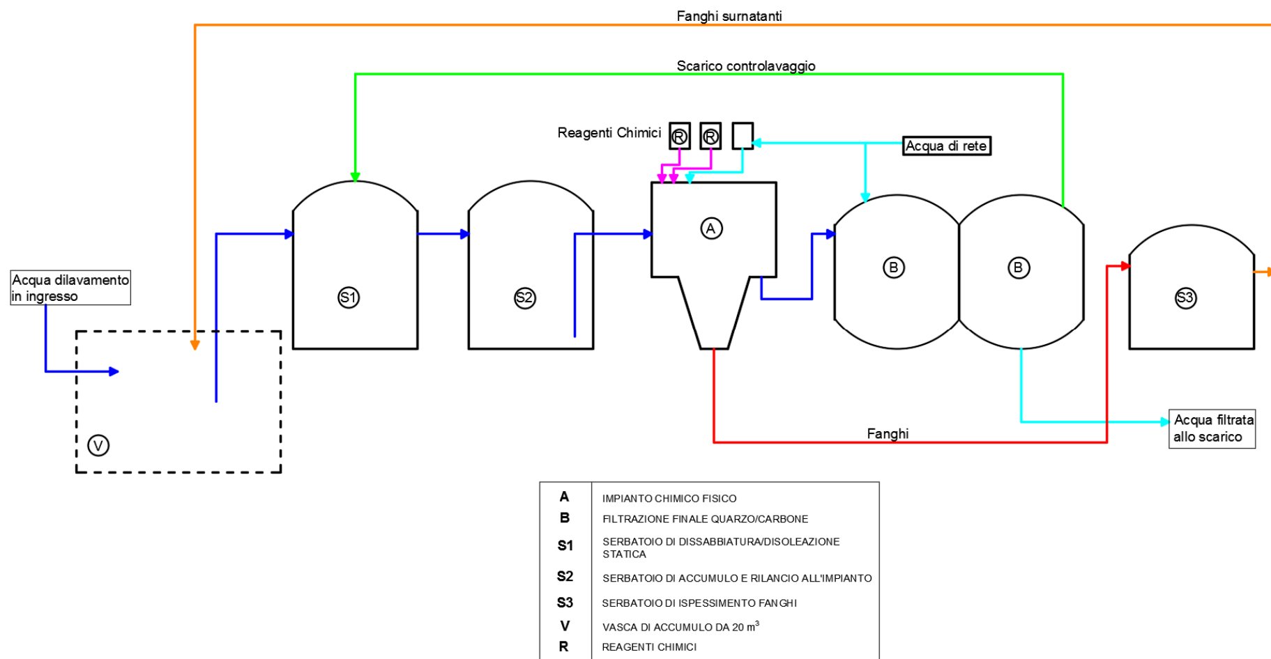
Figura 11 - Schema a blocchi impianto di trattamento chimico-fisico
