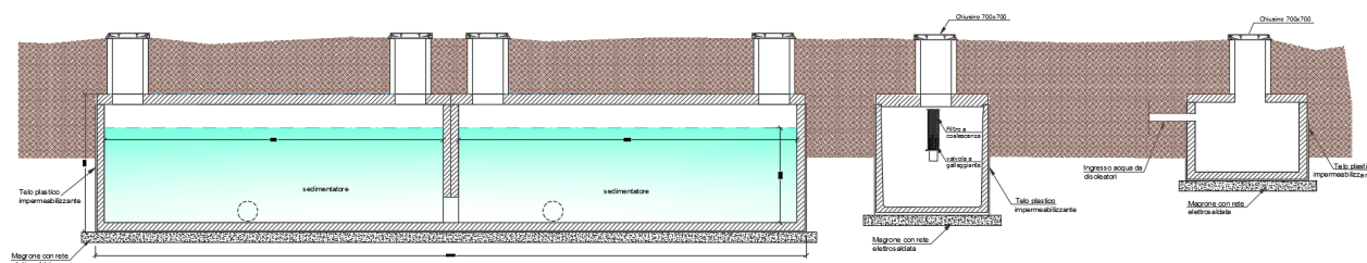
Figura 14 – Sezione di una parte delle nuove vasche
