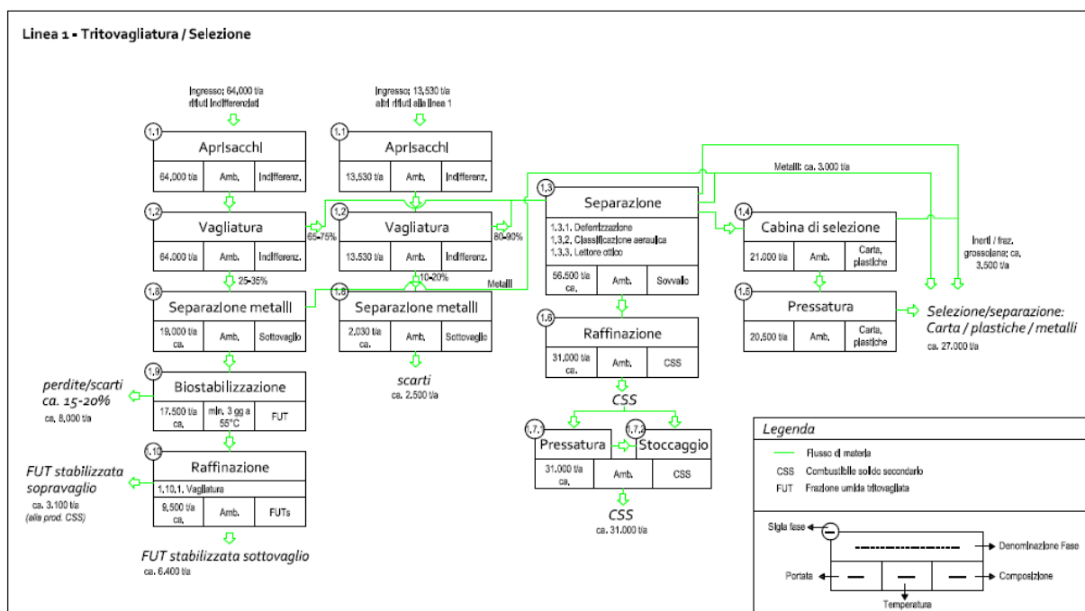
Figura 9 - Schema di flusso quantificato della linea 1
