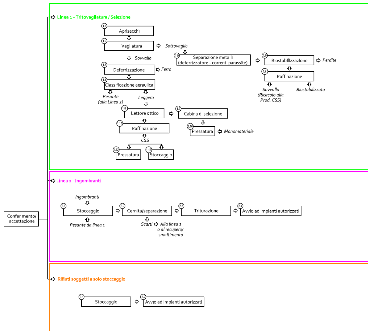
Figura 8 - Schema di flusso generale
