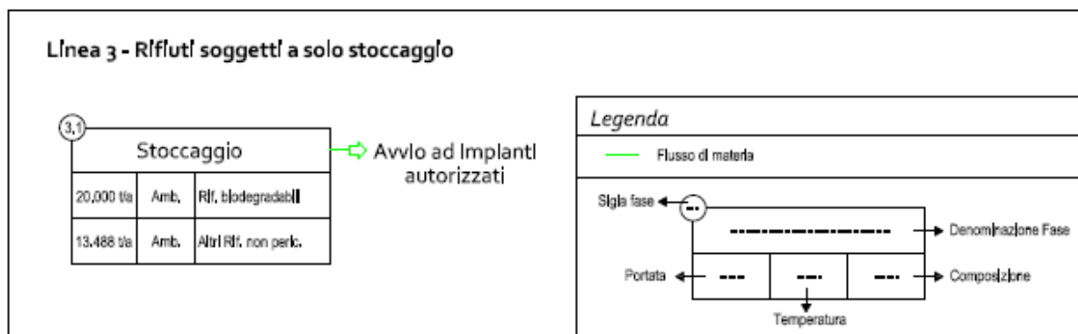
Figura 13 - Schema di flusso quantificato Linea 3
