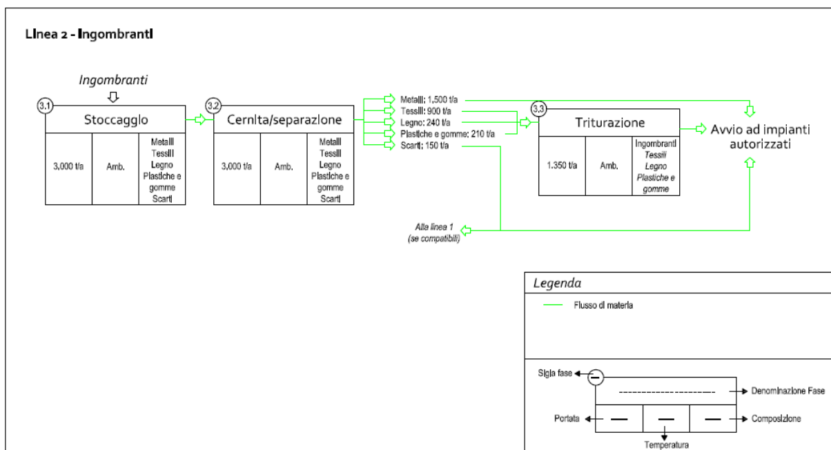
Figura 11 - Schema di flusso quantificato Linea 2
