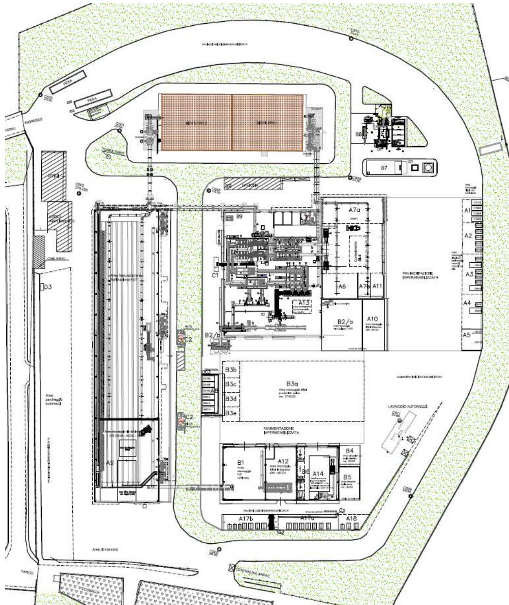
Figura 1 - Lay-out di progetto
