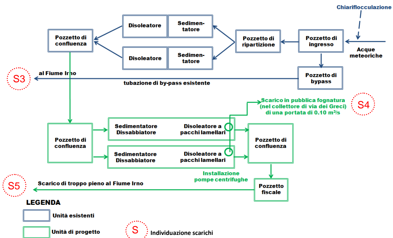
Schema a blocchi impianto di trattamento acque meteoriche
