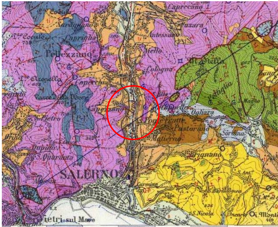
Figura 4.43 - Stralcio della Carta Geologica d'Italia, Foglio 185 Salerno (Scala 1:100000)
