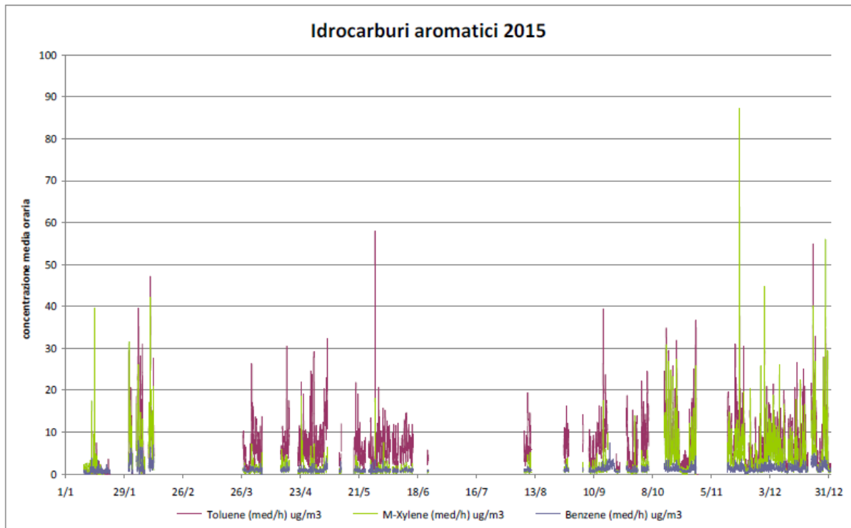
Figura 4.17 - Concentrazioni medie orarie di benzene, toluene e meta-xylene (Relazione ARPAC 2015, fonte www.arpacampania.it )
