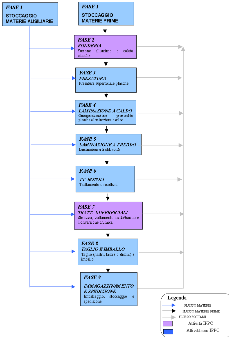
Figura 1 - Schema a blocchi del processo
