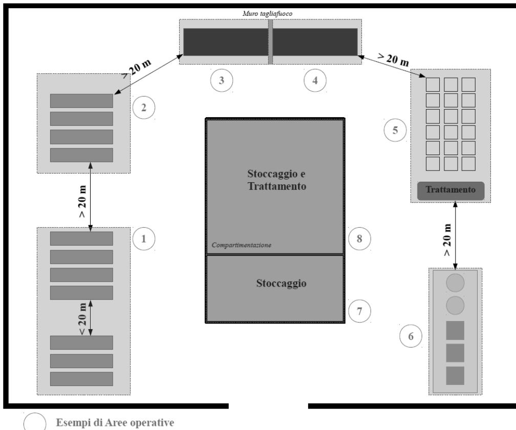
Fig. 2 - Esempio di un impianto di stoccaggio e trattamento rifiuti con aree operative
